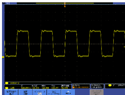
Square 125MHz
