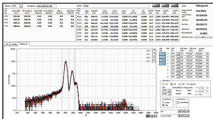
SSD25素子検出器用データ収集システム
